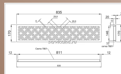
Решетка ВРК-Л Декo «Gotic zvetok», сталь 2мм, сетка ПВЛ 6*4, Ral
