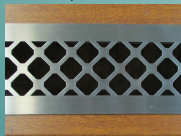
Решетка ВРК-Л «усеченный ромб» Шаг отверстий 20*5мм. Решетка врезная сталь 2мм, Ral.
