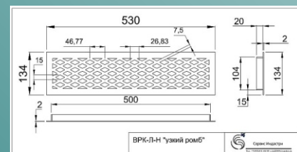
Решетка ВРК-Л «узкий ромб» Решетка врезная сталь 2мм, Ral.
