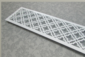
Решетка ВРК-Л Декo «Gotic zvetok», сталь 2мм, сетка ПВЛ 6*4, Ral 9003
