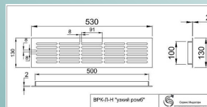
Решетка ВРК-Л «прямо-ник с закру- глением» Шаг отверстий 8*6мм. Решетка врезная ч сталь 2мм. Ral.
