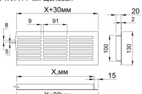
ВРК-Л-Н 7-ми щелевая
