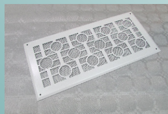
Решетка ВРК-Л Архитектурная «Круги в рамках», сталь 2мм, Ral 9003, сетка ПВХ 6*4
