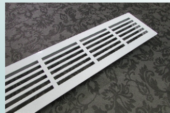
Решетка ВРК-Л «прямоугольник» Шаг отверстий 8*6мм. Решетка врезная сталь 2мм, Ral
