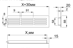
ВРК-Л-Н 4-х щелевая
