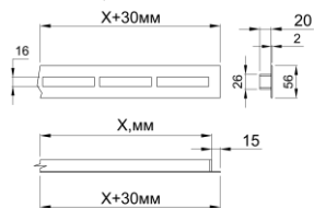
ВРК-Л-Н 1-на щелевая
