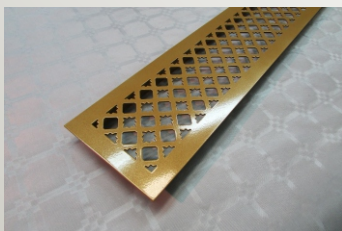
Решетка ВРК-Л Декo «Звездное небо», сталь 2мм, сетка ПВЛ 6*4, Ral 1036
