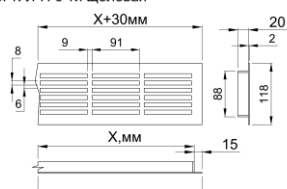
ВРК-Л-Н 6-ти щелевая
