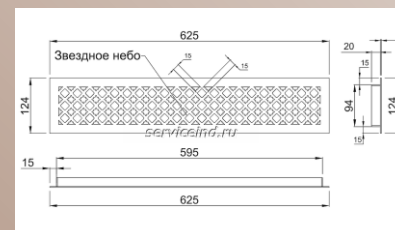
Решетка ВРК-Л Декo «Звездное небо», сталь 2мм, сетка ПВЛ 6*4, Ral
