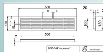
Решетка ВРК-Л «Кирпичик» Шаг отверстий 8*6мм. Решетка врезная сталь 2мм, Ral
