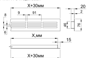
ВРК-Л-Н 3-х щелевая
