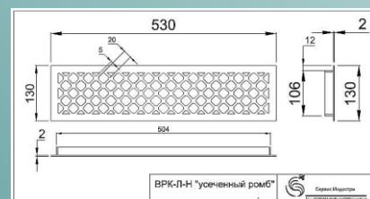
Решетка ВРК-Л «усеченный ромб» Шаг отверстий 20*5мм. Решетка врезная сталь 2мм, Ral.
