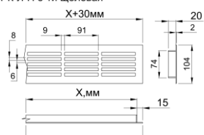
ВРК-Л-Н 5-ти щелевая
