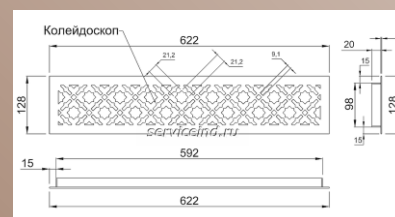
Решетка ВРК-Л Декo «Колейдоскоп», сталь 2мм, сетка ПВЛ 6*4, Ral 1015
