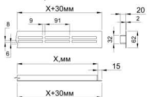
ВРК-Л-Н 2-х щелевая
