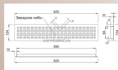
Решетка ВРК-Л Декo «Звездное небо», сталь 2мм, сетка ПВЛ 6*4, Ral
