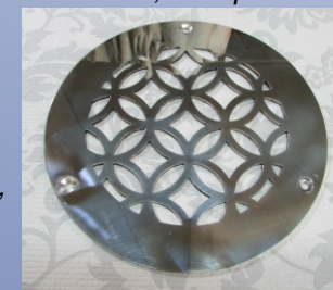
«Круги» D-150, нерж сталь 2мм, полировка
