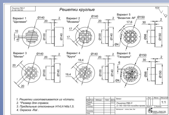
Решетки ВРК-Л «Круглые D-100*»
