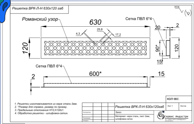
Решетка ВРК-Л-Н «Романский узор»
