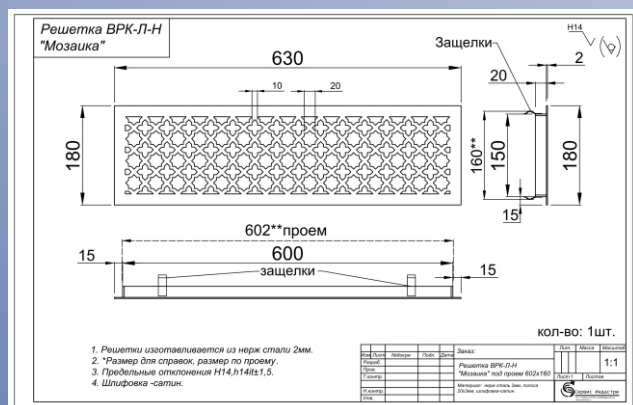
Решетка ВРК-Л-Н «Мозаика»
