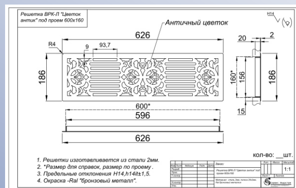
Решетка ВРК-Л «Античный цветок»
